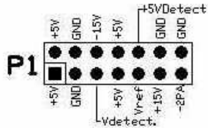
Vista lato componenti SMD
