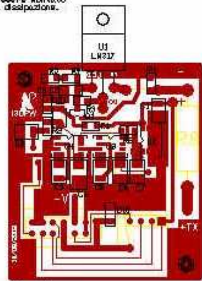
Vista lato componenti SMD
